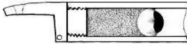
Dwarsdoorsnede hoe de kruitlading en de kogel in de loop zaten.
